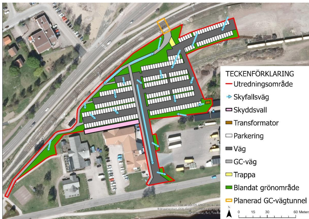
Figur 20. Föreslagna framtida skyfallsvägar och skyddsvall inom utredningsområdet.
