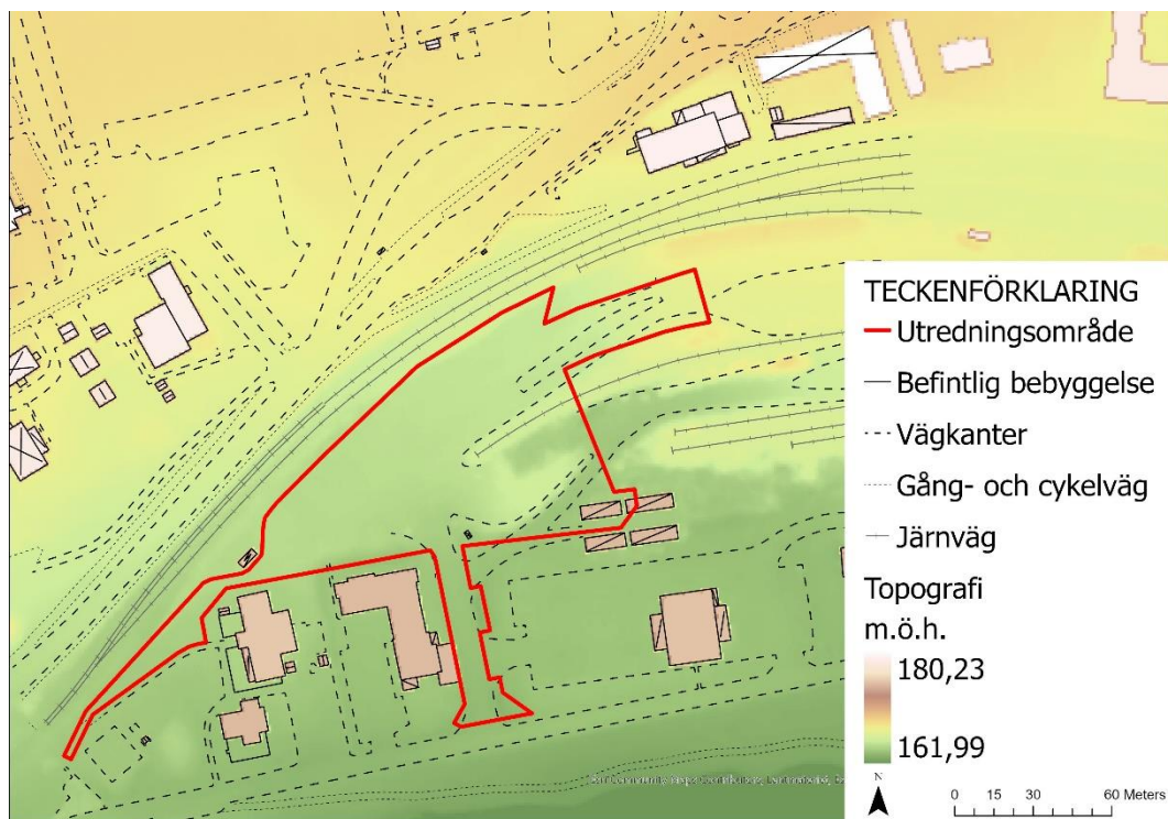
Figur 3. Befintlig topografi inom och utanför utredningsområdet (SCALGO, 2023).
