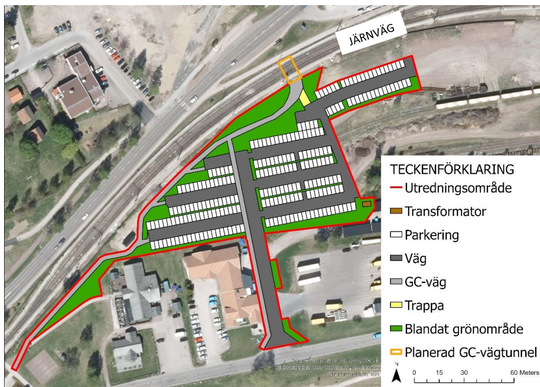
Figur 15. Ungefärlig utformning av det framtida utredningsområdet.
