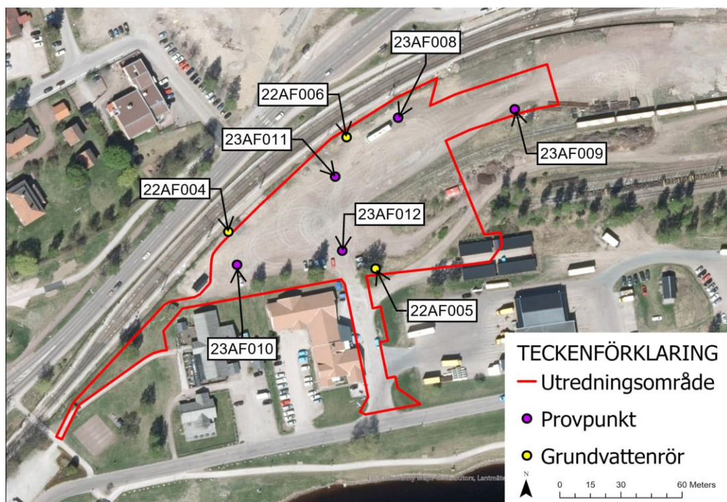
Figur 7. Placering av installerade grundvattenrör och provpunkter för provtagning av jord (AFRY, 2024b; AFRY, 2024c).
