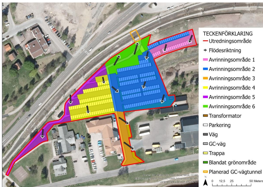
Figur 16. Antagna avrinningsområden för det framtida utredningsområdet.
