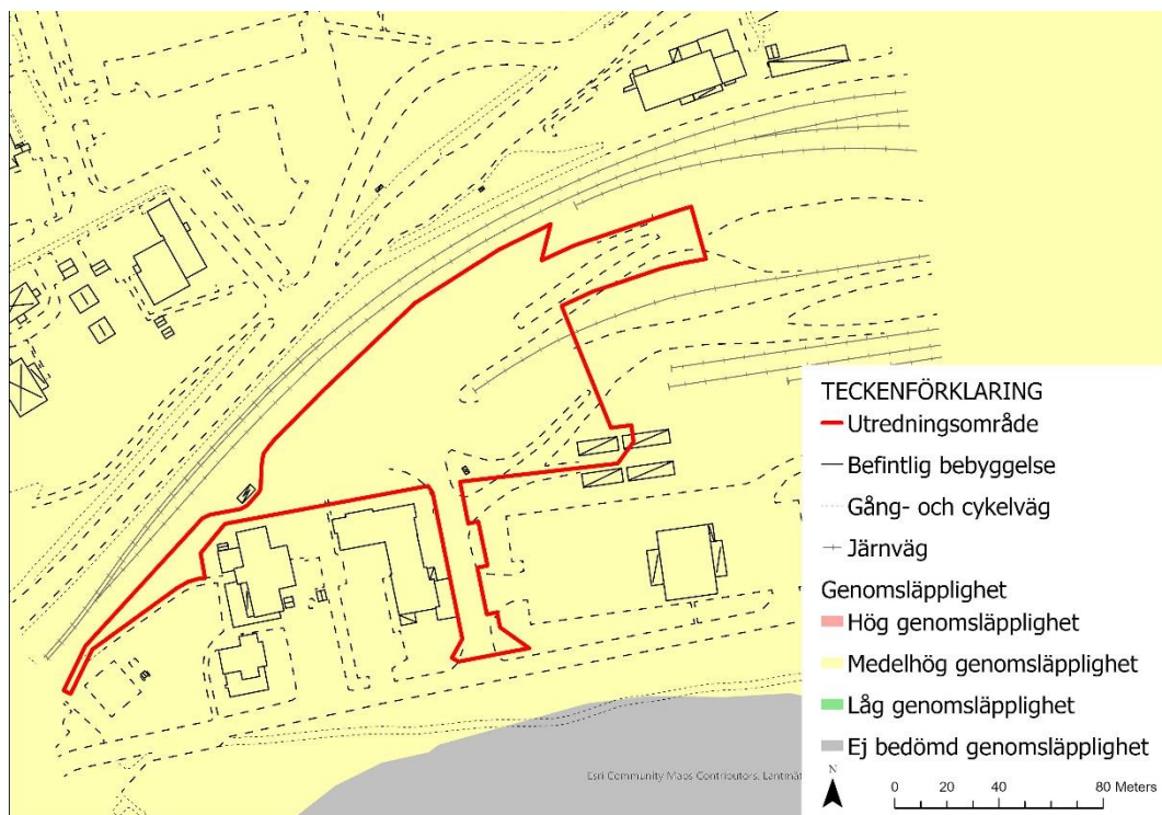
Figur 6. Genomsläppligheten inom utredningsområdet är medelhög (SGU, 2023c).
