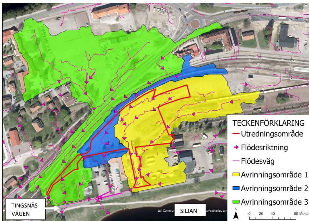
Figur 10. Befintliga avrinningsområden och flödesvägar (SCALGO, 2023).
