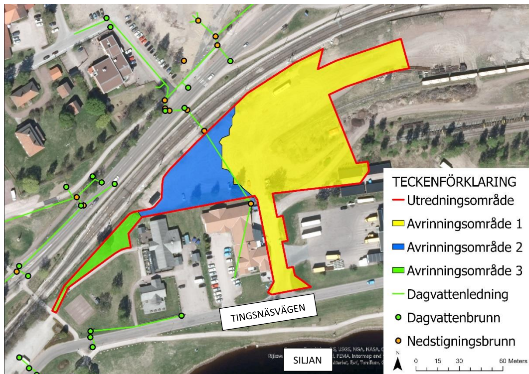
Figur 11. Befintligt dagvattenledningsnät och avrinningsområden (SCALGO, 2023).
