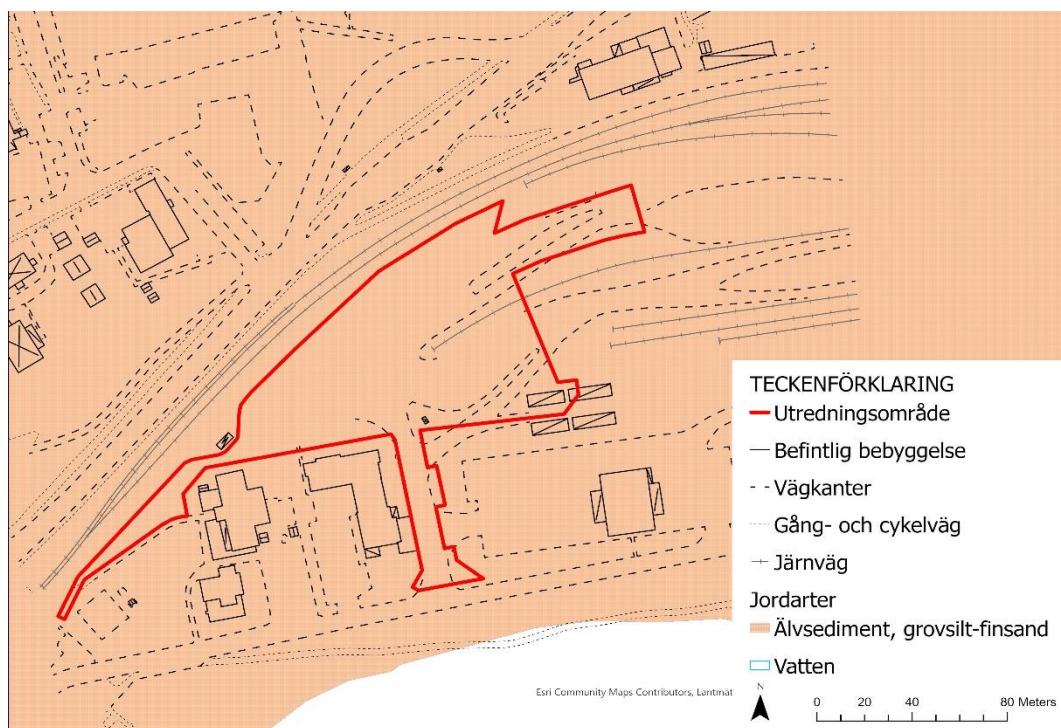
Figur 4. Jordarten inom och utanför utredningsområdet är älsediment (SGU, 2023a).
