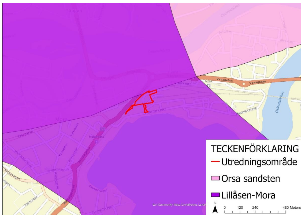
Figur 9. Ungefärlig utbredning av grundvattenförekomsterna (VISS, 2021b; 2021c).
