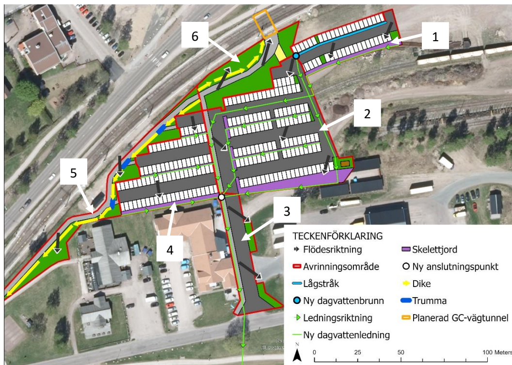
Figur 17. Förslag till hantering av dagvatten inom vardera avrinningsområde för det framtida utredningsområdet.
