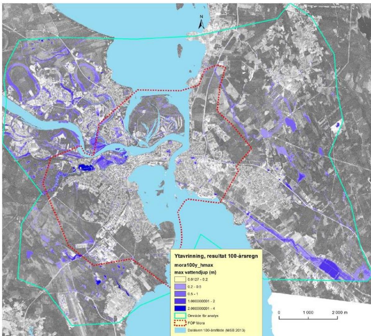
Figur 2. Ytavringning vid 100-årsregn (lila, mörkare färg innebär större potentiellt vattendjup). Bilden visar även MSB:s översvänningskartering av 100-årsflöde i Dalälven (ljusblå färg).
